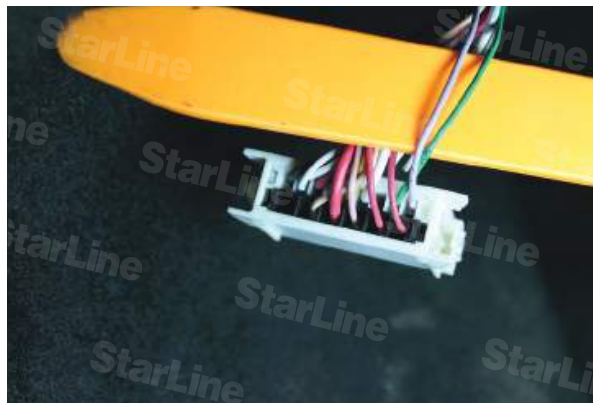
Фото 10.2. Поворотники-фиолетовый и зеленый (белый разъем блока ВСМ)
